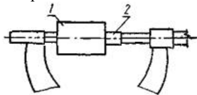
1 - концевая мера длины; 2 - динамометр Рис. 1.
